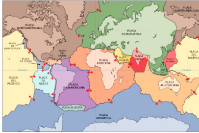
Figura 13. Placas tectónicas.
