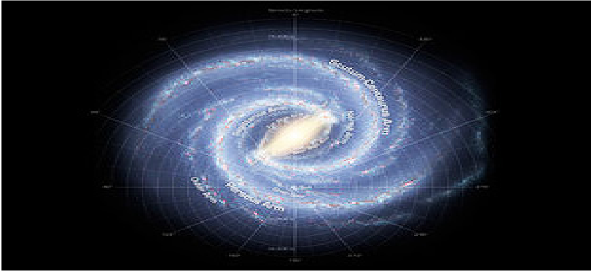
Figura 7. Vía Láctea
